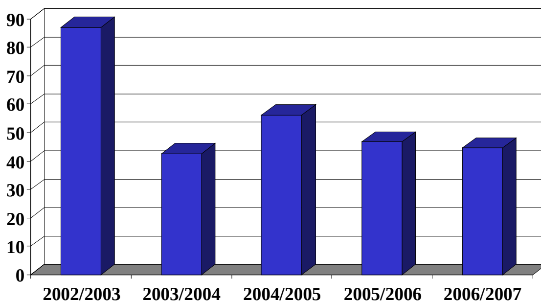
Figure 27 – Productions de civelles en tonnes sur la façade maritime française par les marins-pêcheurs au cours des cinq dernières années (Source : SIH, Etude socio-économique de la pêche cavière française, IFREMER 2008)
