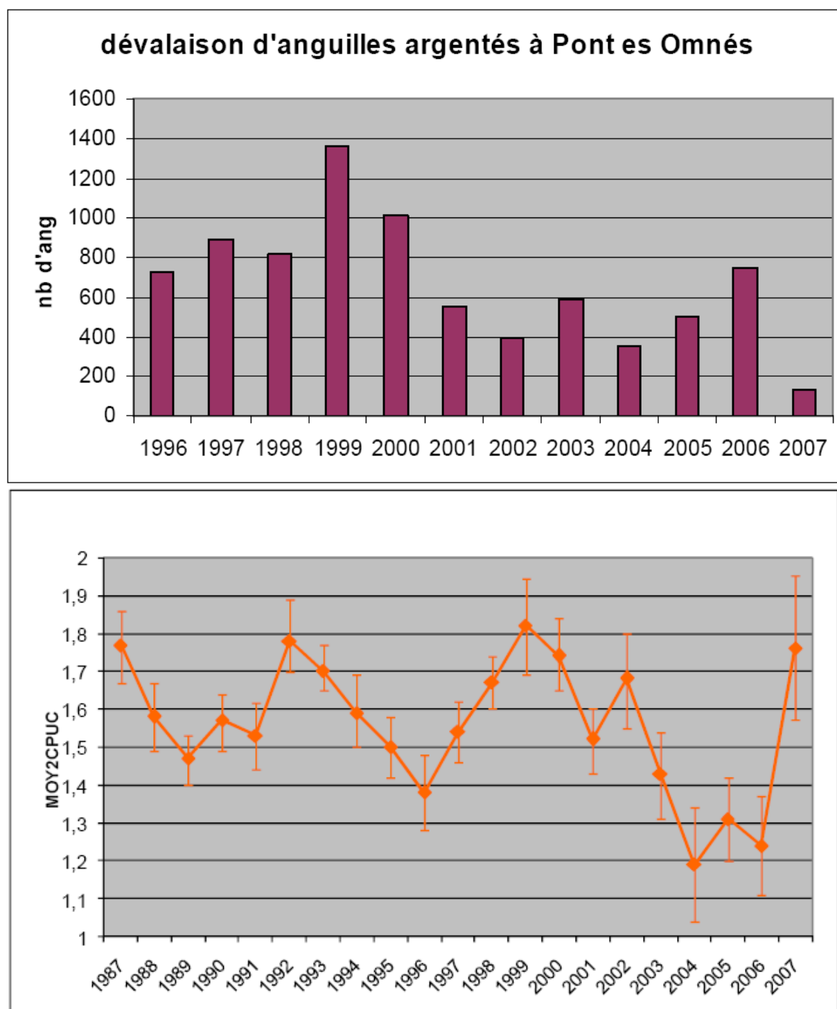
Figure 6 : Nombre d'anguilles dévalant à Pont es Omnés sur le Frémur (haut, source Ouest Grand Migrateur) et indice d'abondance de la pêche d'argentées de la Loire (bas, Bodin et al., 2008)
