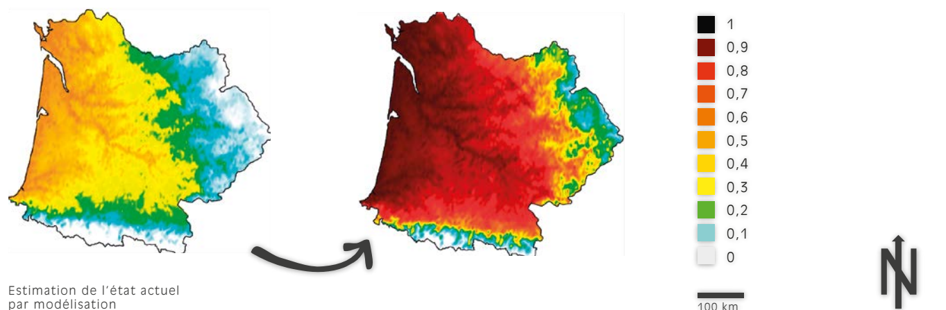
Évolution probable de la Jussie, plante aquatique invasive représentative de 38 espèces végétales thermophiles étudiées sur le bassin (D'après E. Tabbachi, non encore publiés)
