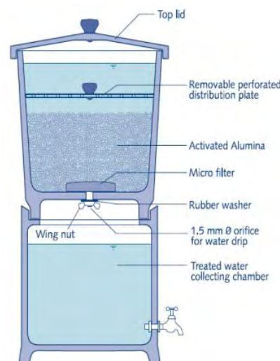
Figure 13 : Vue en coupe d'un filtre à alumine activée
