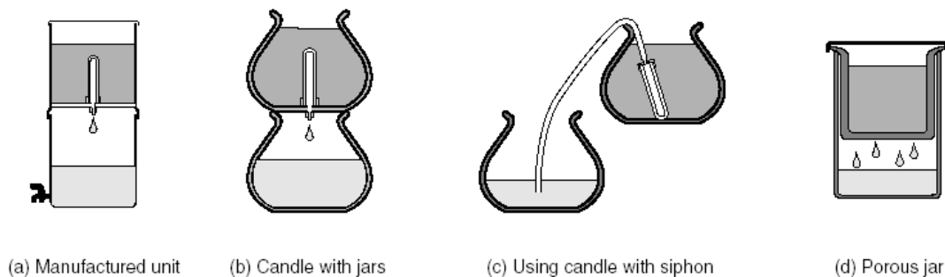
Figure 7 : Différents modèles de filtres en céramique
