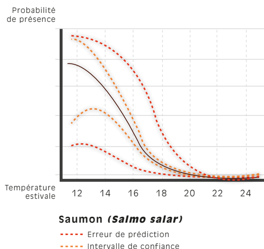
Profils marginaux de probabilité de présence pour les espèces saumon et ablette en fonction des températures estivales de l'eau (Adapté de BASILICO et al., 2009)
