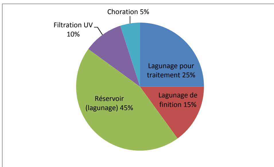
Figure 14 : Type de désinfection utilisées (enquête Irstea-SATESE 2011)
