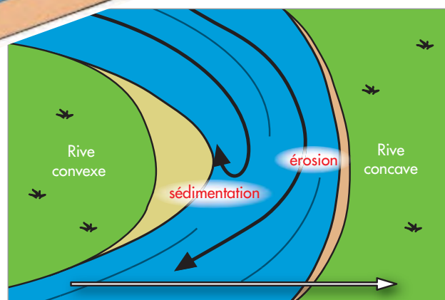
▲ Méandriformes
