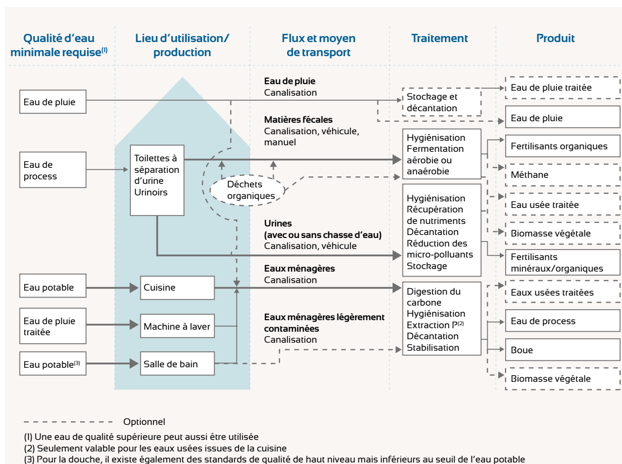
FIGURE 4 Exemple de séparation à la source : système à trois flux avec séparation des urines (toilettes à séparation). Cf. cas n°5 dans la figure 2. (Pour aller plus loin, voir DWA, 2010).
