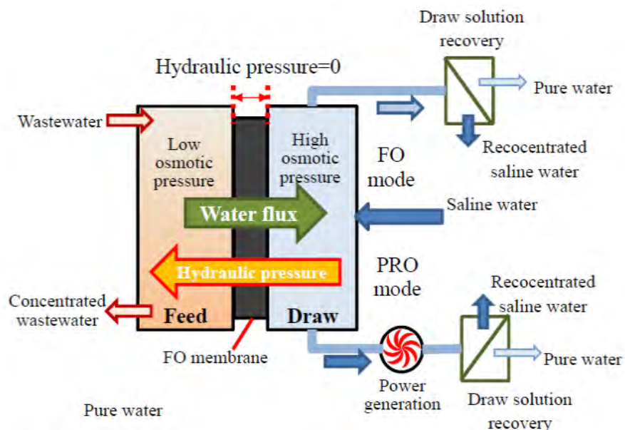
Figure 10: Principe de fonctionnement de l'osmose directe (Lu et al., 2015)
