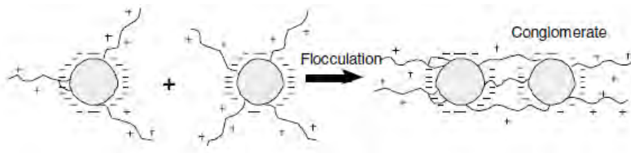
Figure 2: Principe de la floculation: cas d'un chlorure de polyaluminium (Lens et al., 2002)
