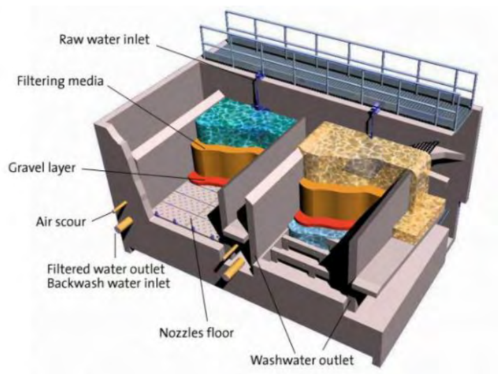
Figure 6: Schéma type d'une filtration sur média filtrant (Veolia)
