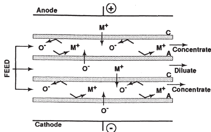
Figure 12: Principe de fonctionnement de l'électrodialyse (Scott & Hughes, 2012)
