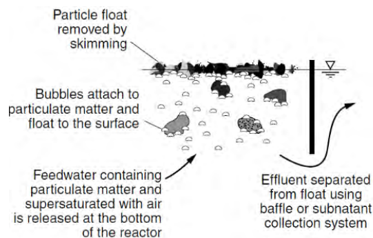
Figure 5: Principe de fonctionnement d'une Flottation à Air Dissous (Asano et al., 2007)
