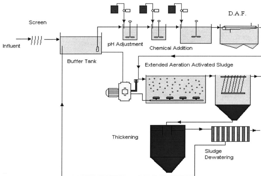
Figure 17: Schéma de la station d'épuration des eaux usées d'une industrie de raffinage d'huile végétale dans la ville de Bursa, Turquie (Azbar & Yonar, 2004)
