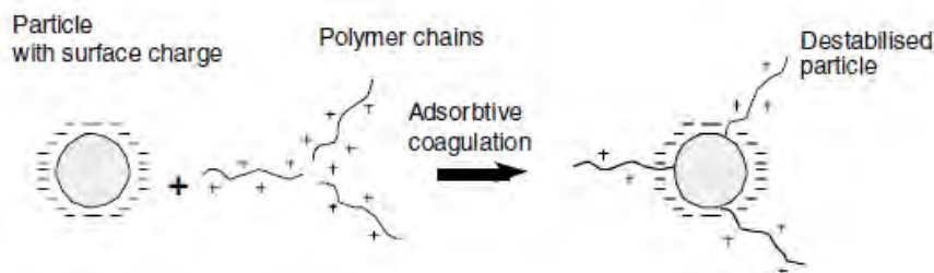
Figure 1: Principe de la coagulation : cas d'un chlorure de polyaluminium (Lens et al., 2002)
