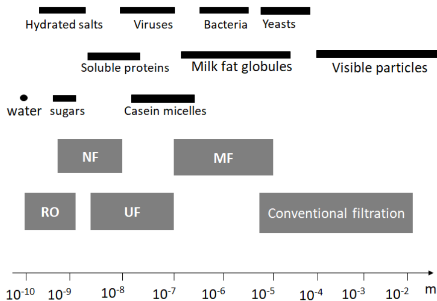
Figure 8: Taille des différents solutés comparée au diamètre des pores
