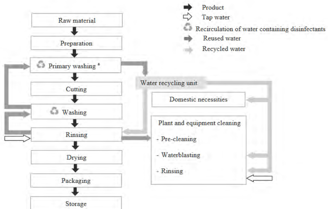
Figure 16: Solutions de réutilisation et de recyclage pour une industrie de conditionnement de jeunes pousses de salade (Manzocco et al., 2015)
