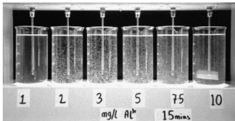
Figure 3: Exemple de jar-test (Parsons & Jefferson, 2006)
