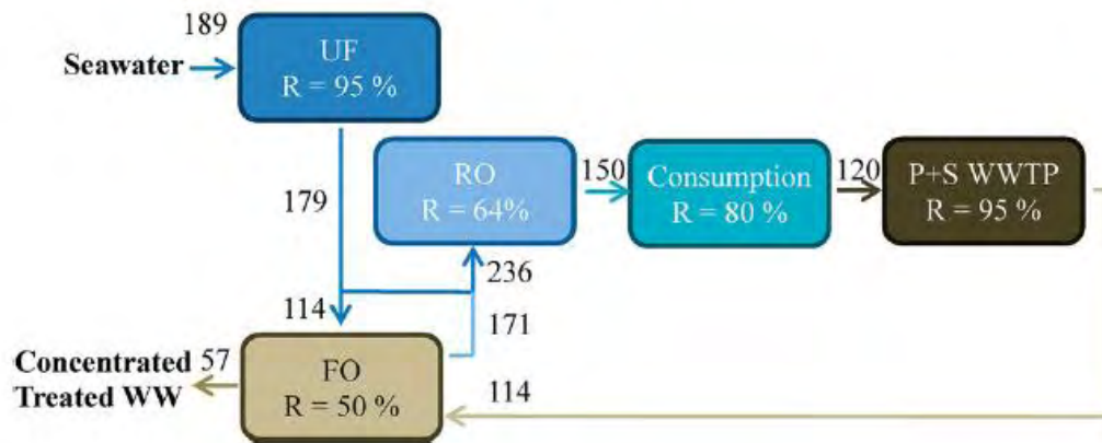
Figure 15: Principe de la combinaison de la réutilisation des eaux usées et du dessalement de l'eau de mer (Teusner et al., 2017)
