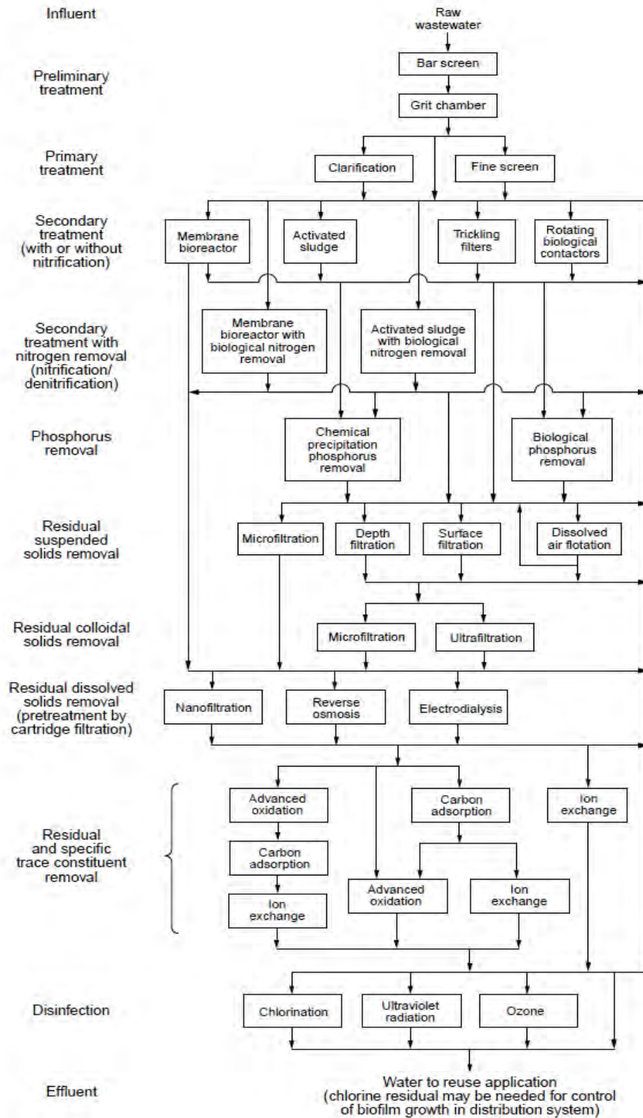
Figure 18: Disposition hiérarchique des technologies de traitement possibles (Asano et al., 2007)
