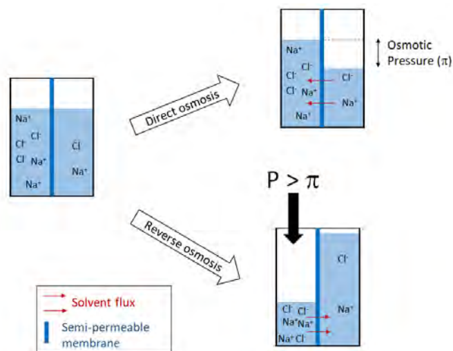
Figure 9: Principe de fonctionnement de l'osmose inverse et de l'osmose directe
