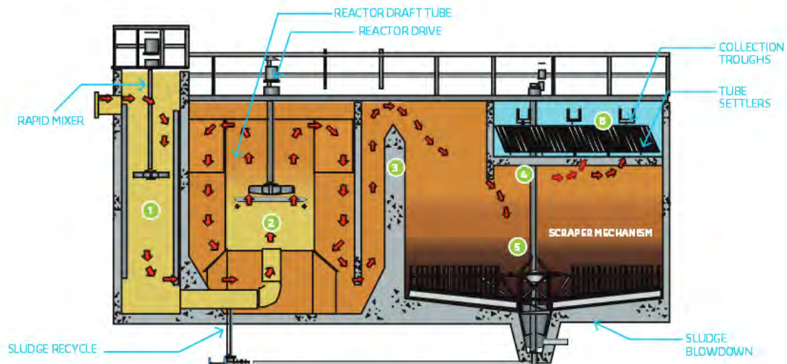
Figure 4: Schéma type d'une unité de coagulation, floculation et décantation (Degrémont)
