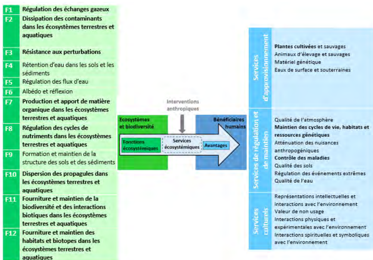
Figure 4. Liens entre fonctions et services écosystémiques (en gras : fonctions et services documentés dans le corpus bibliographique, en lien avec les PPP). Adapté d'EFSE 2016 1 .
