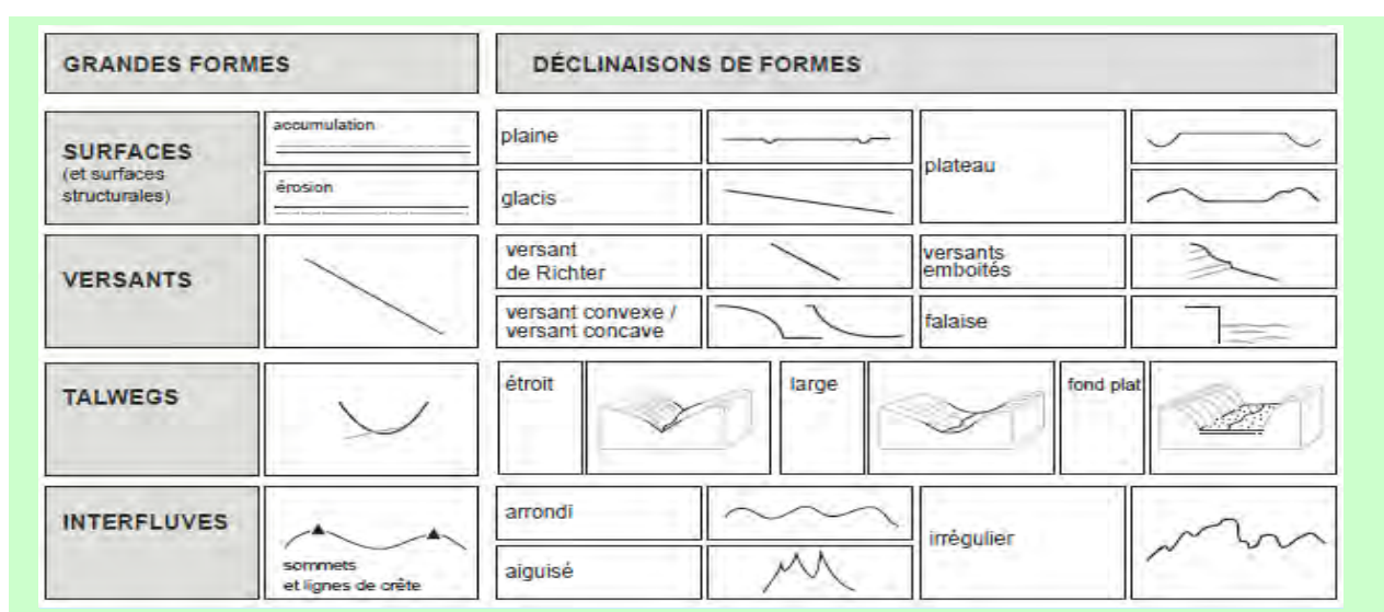
Figure 15 : illustration de grandes entités géomorphologiques et des formes du relief associées (Claire PORTAL. 2010).
