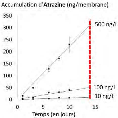
Fig. 32. Expérience d’accumulation d’Atrazine sur des chemcatchers. Durée d’incubation maximale de 15 jours, pour 3 concentrations d’Atrazine (Pinasseau et al. 2020 dans Talanta).
