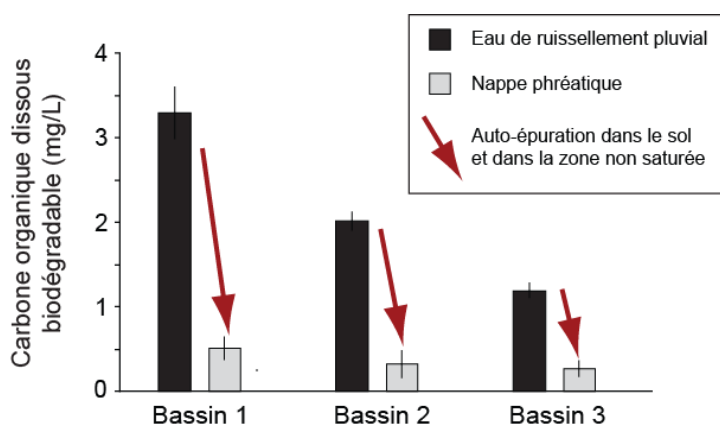
Fig. 16. Teneurs en fraction biodégradable du carbone organique dissous dans les eaux de ruissellement et dans la nappe située en dessous de 3 bassins d'infiltration de la métropole de Lyon ( Mermillod-Blondin et al. 2015 dans Water Research)
