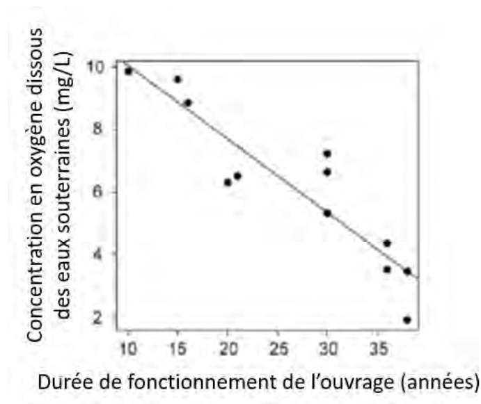
Fig. 26. Relation entre l'Oxygène dans la nappe et l'âge de 12 bassins d'infiltration de la Métropole de Lyon (Foulquier 2009).
