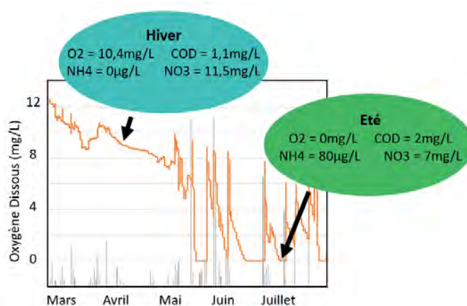
Fig. 28. Suivi en continu des teneurs en oxygène dissous et mesures ponctuelles des nutriments en aval du bassin de l'IUT à la Doua (données OTHU 2017)
