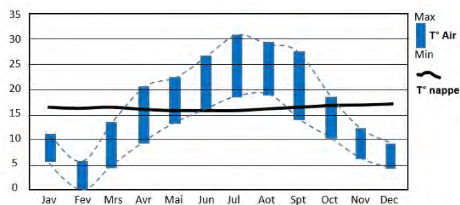
Fig. 2. Température de la nappe comparée à celle de l'air (en minimum-maximum mensuels, données Météo-France).
