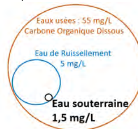
Fig. 3. Teneurs moyennes en carbone organique dissous dans trois types d'eau
