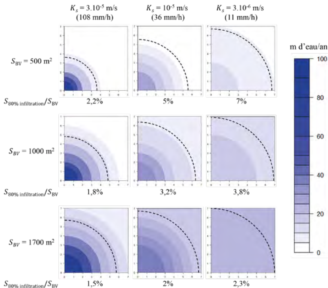
Figure 8.2 – Lamé d'eau infiltrée (exprimée en mètres d'eau par an) dans les différentes zones d'un espace de 50 m 2 sans exutoire, en fonction de la perméabilité du sol K_s et de la surface du bassin versant S_{BV} . La courbe en pointillés délimite la zone où s'infiltré 80% de la pluie totale.
