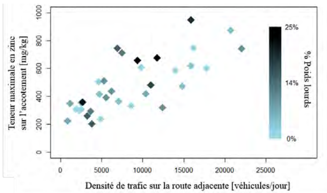
Figure 9.1 – Teneurs maximales en zinc mesurées sur des accotements routiers, représentées en fonction de la densité de trafic sur la route adjacente.
